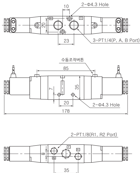
2위치 / 5포터 더블형(그로맷 타입)
