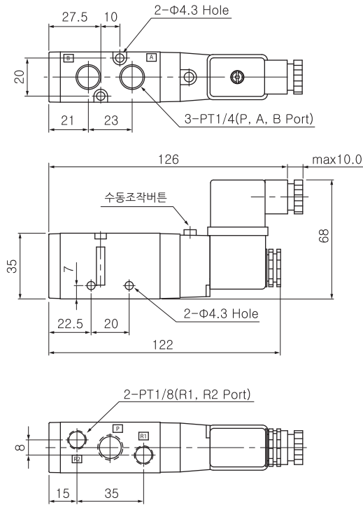
2위치 / 5포터 싱글형(커넥터 타입)
